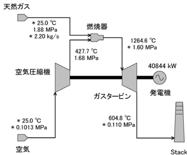
EnergyWinで作成した、単純ガスタービンサイクルの解析用系統図
